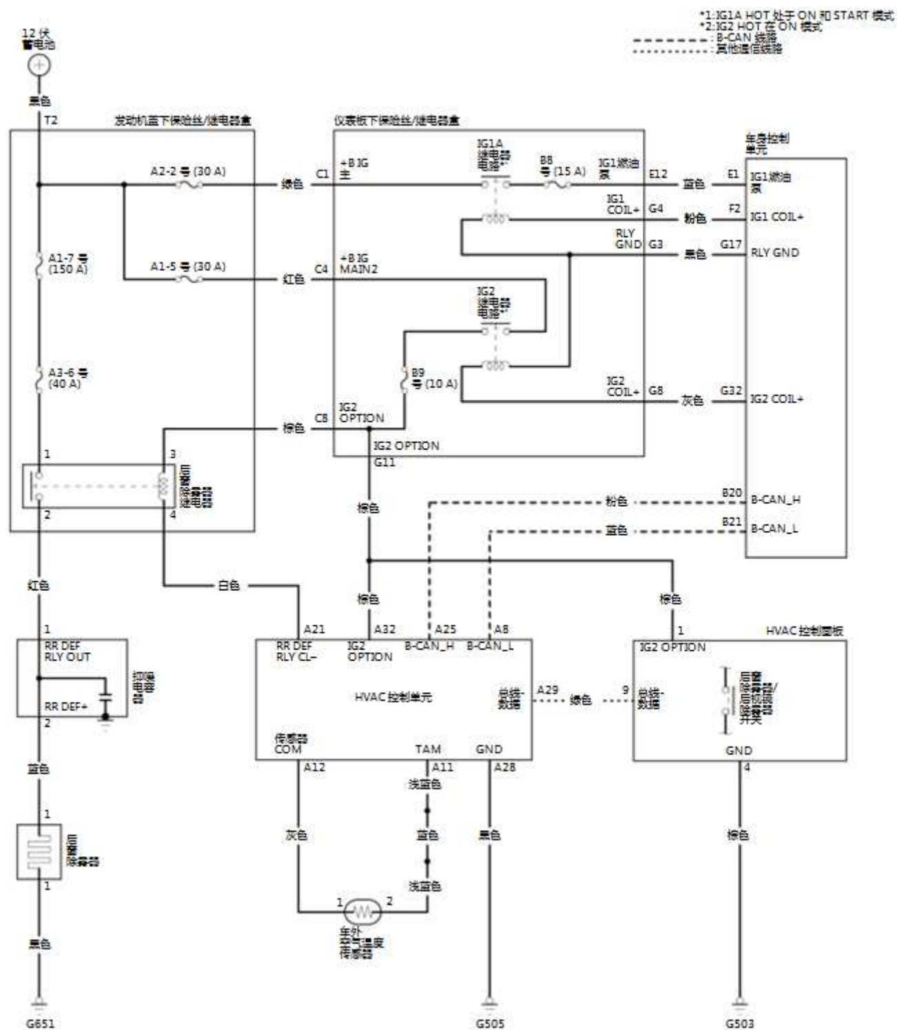
后窗除雾器电路图
